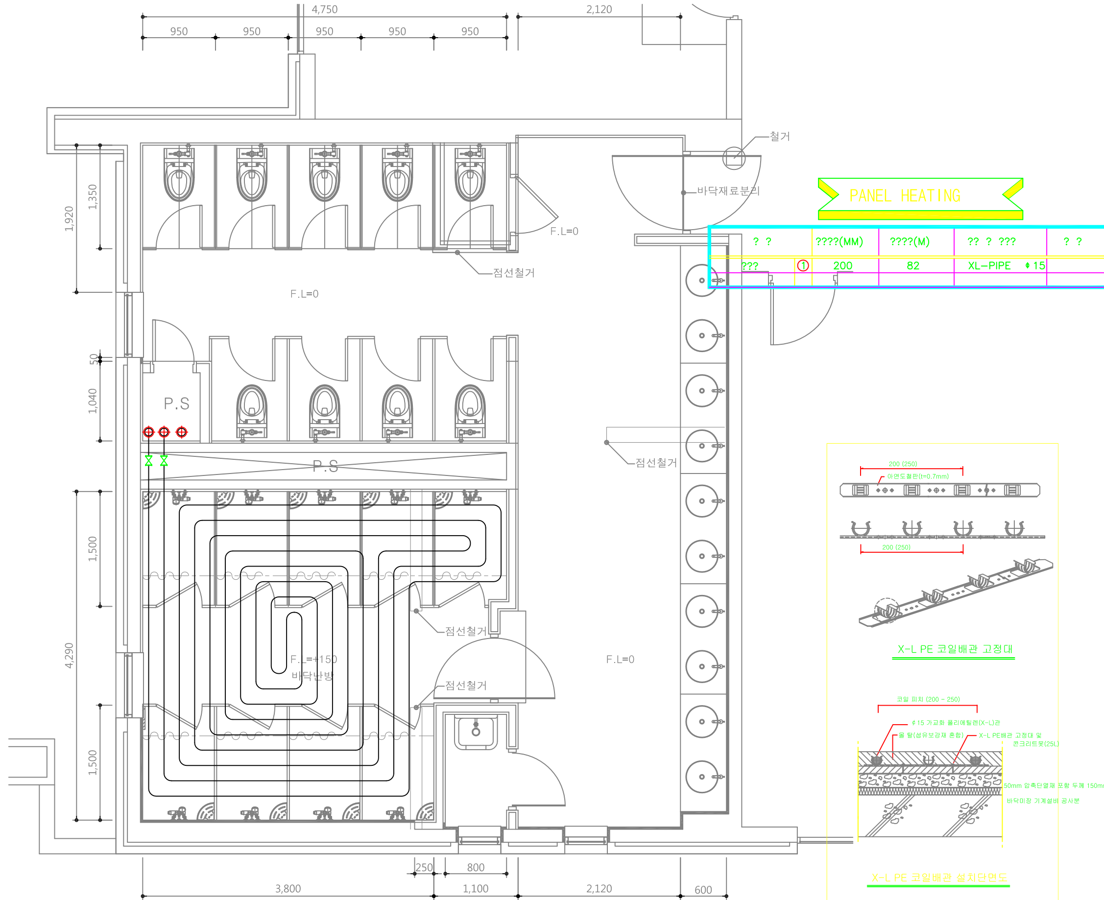
2,3,4층 화장실 확대 난방배관 평면도(서북측)
