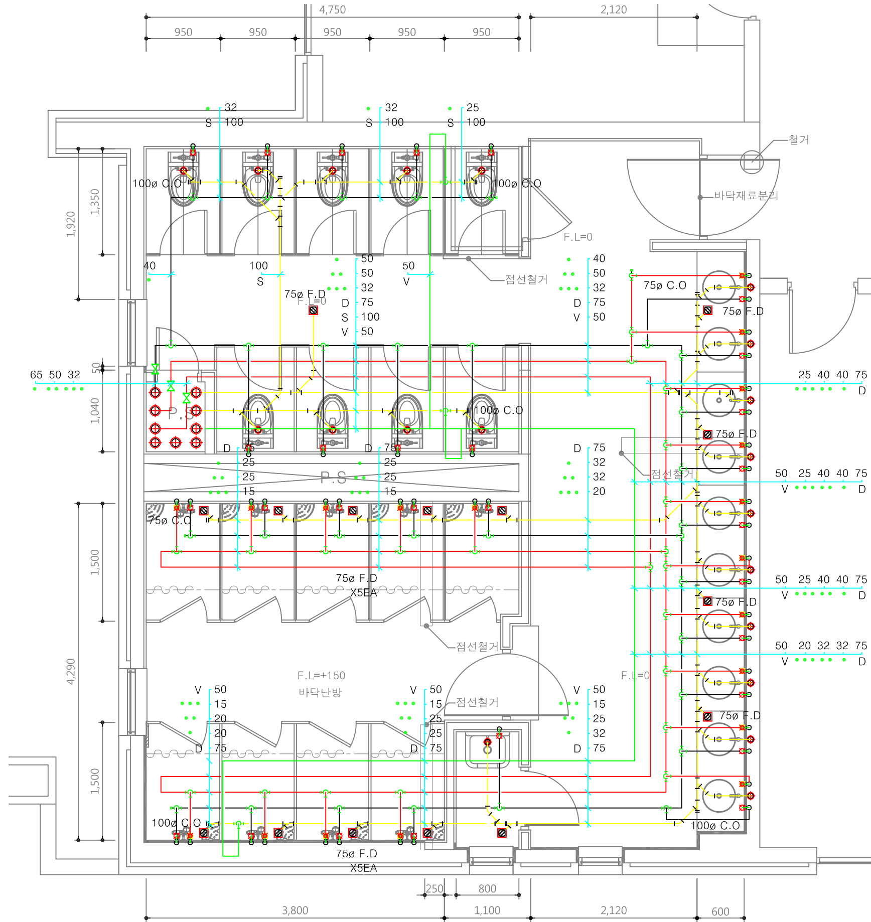
2,3,4층 화장실 확대 위생배관 평면도(서북측) 축척 = (A1)1/ 25 (A3)1/ 50
