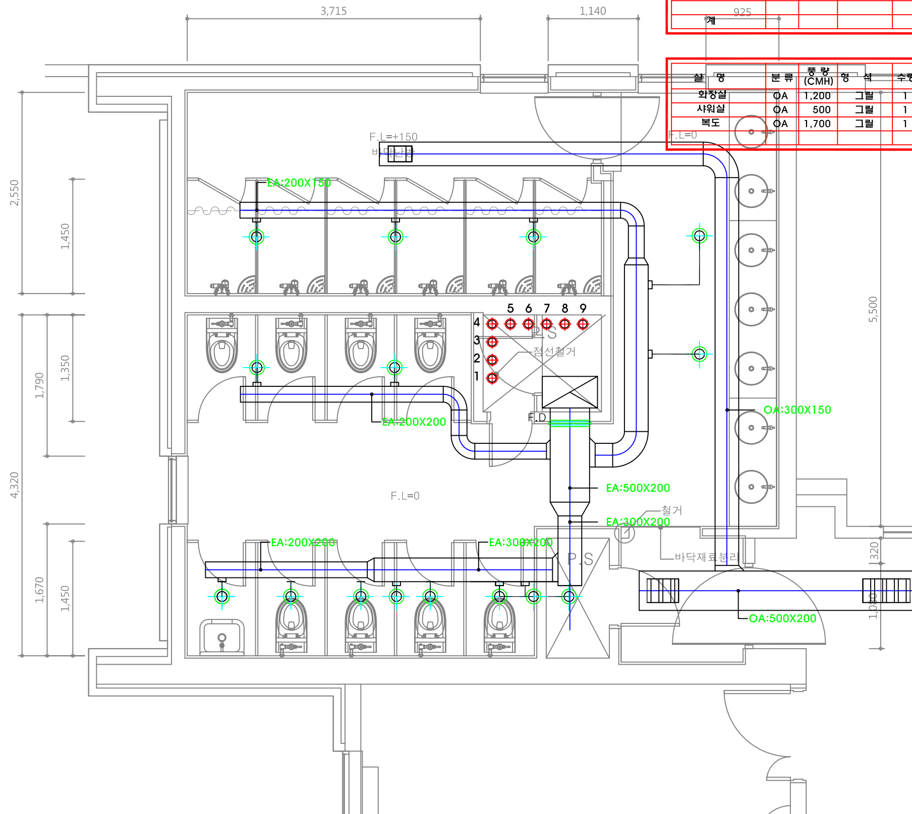
4층 화장실 확대 환기덕트 평면도(동북측) 축척 = (A1)1/25 (A3)1/50
