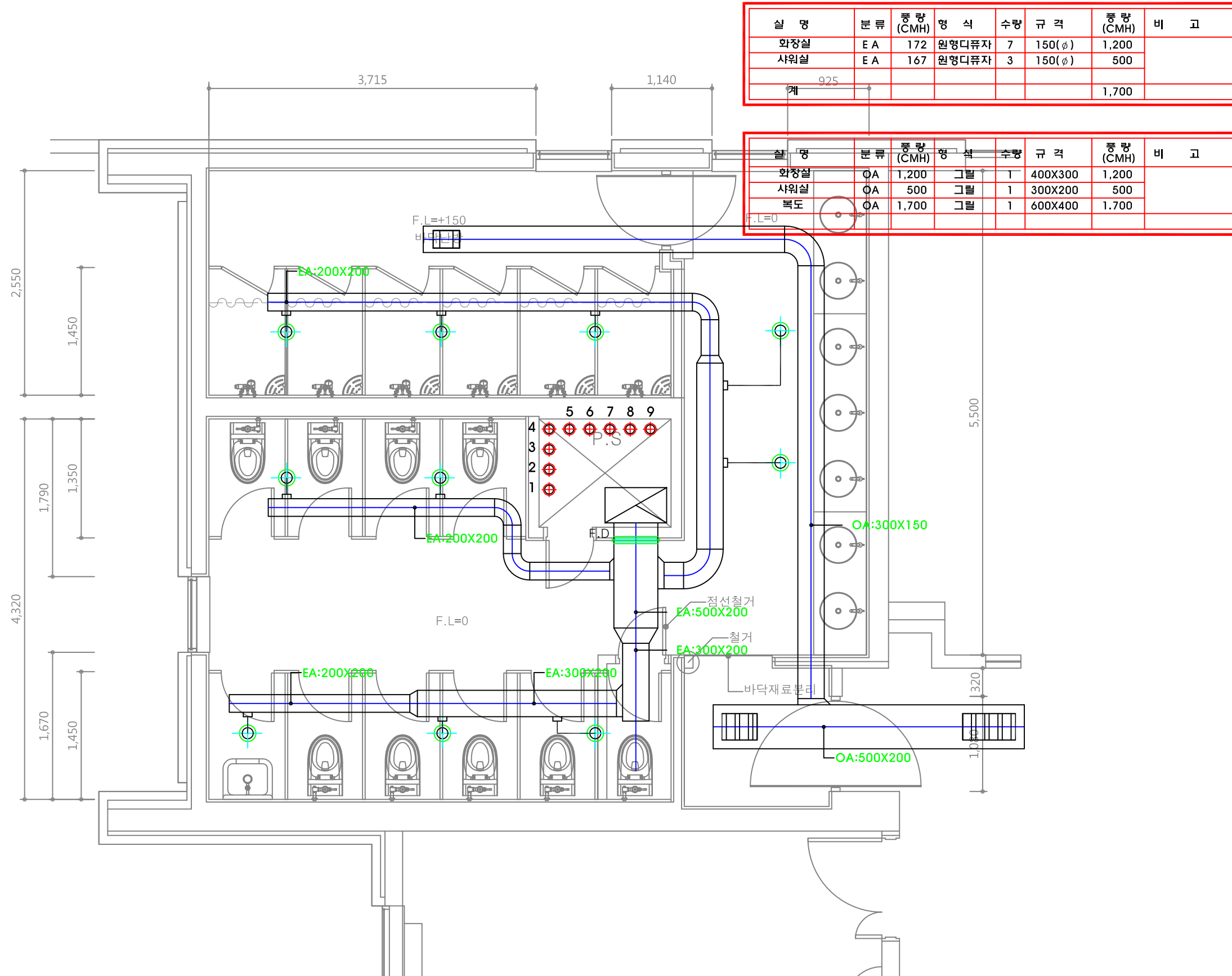
2,3층 화장실 확대 환기덕트 평면도(동북측)
