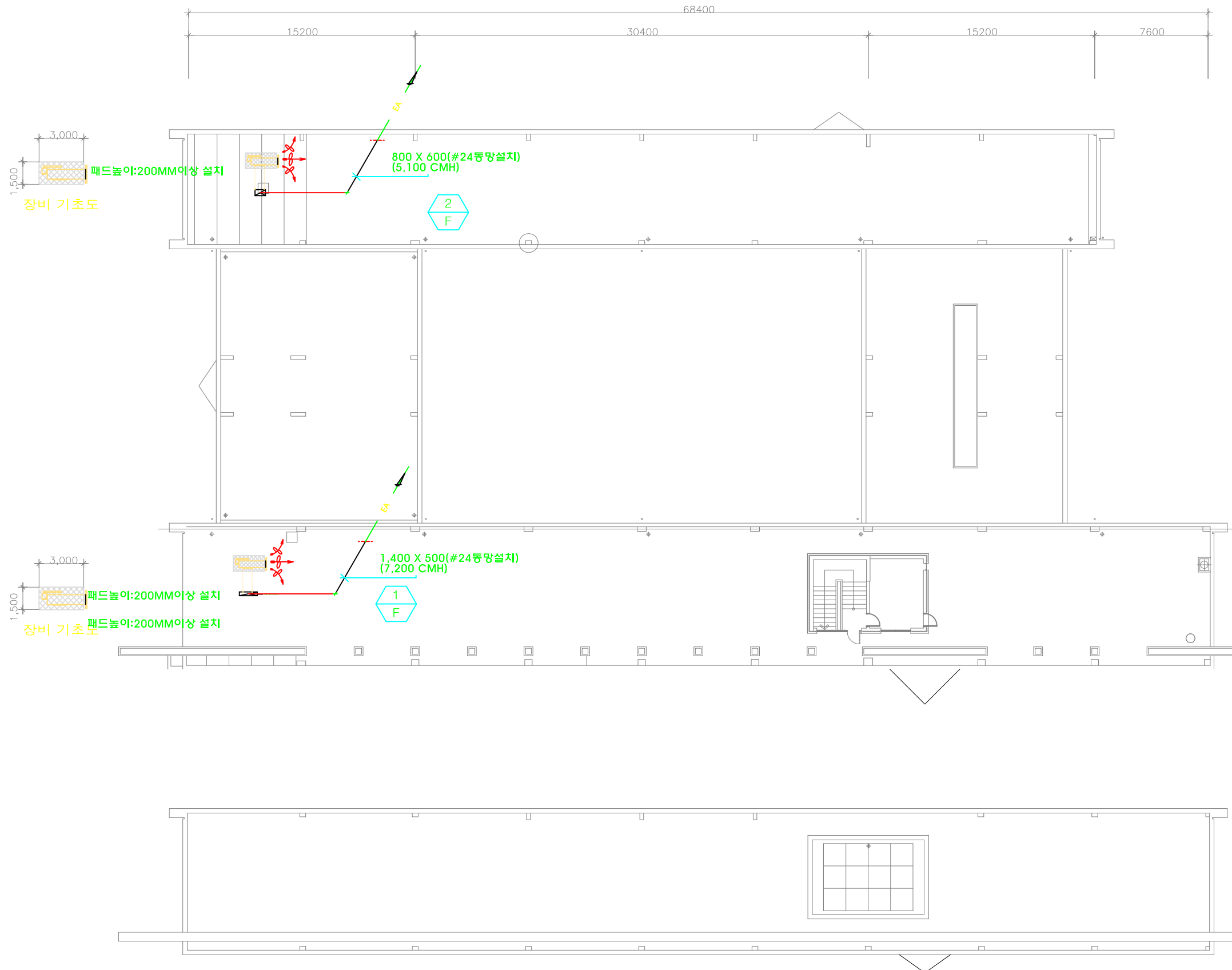
지붕층 환기덕트 평면도 축척 = (A1) 1/150 (A3) 1/300
