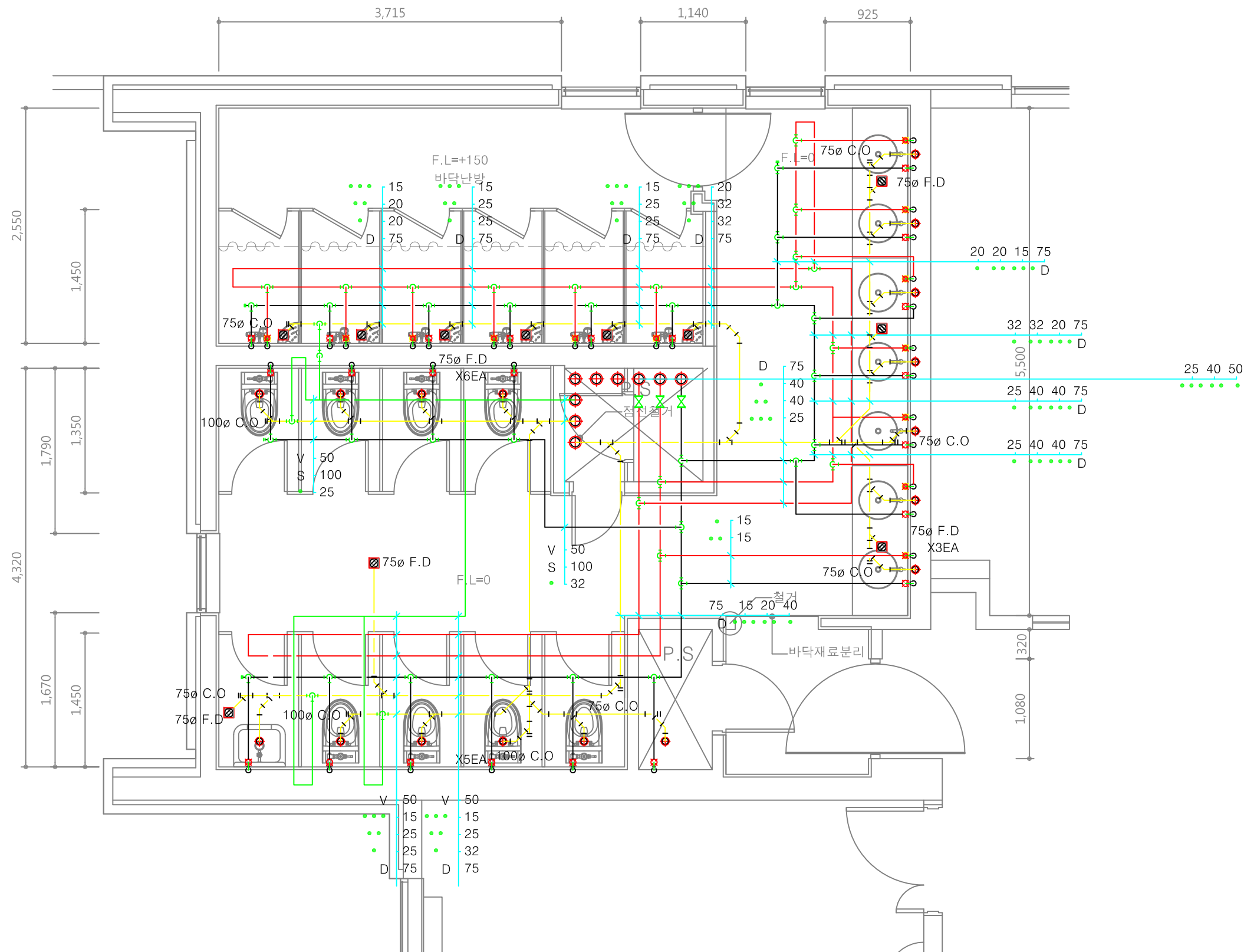
4층 화장실 확대 위생배관 평면도(동북측) 축척 = (A1) 1/25 (A3) 1/50
