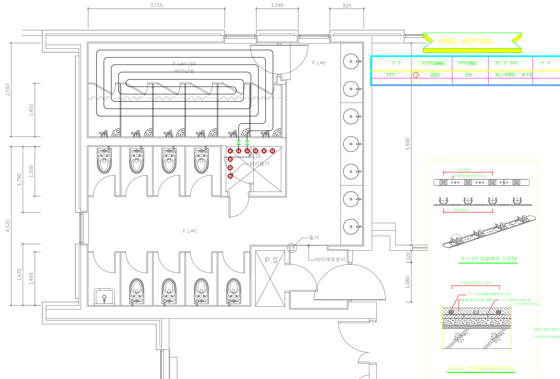
1 M 4층 화장실 확대 난방배관 평면도(동북측) 축척 = (A1)1/ 25 (A3)1/ 50
