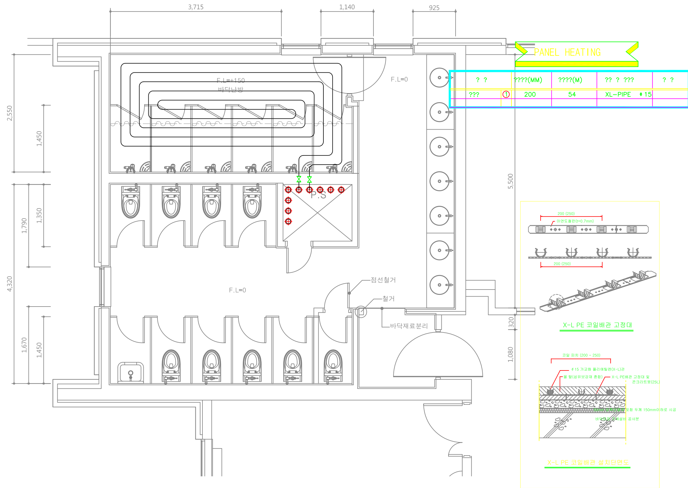
2,3층 화장실 확대 난방배관 평면도(동북측)
