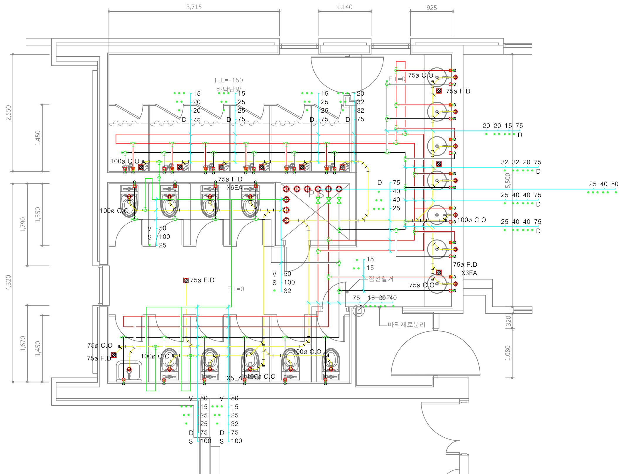
2,3층 화장실 확대 난방배관 평면도(동북측)
