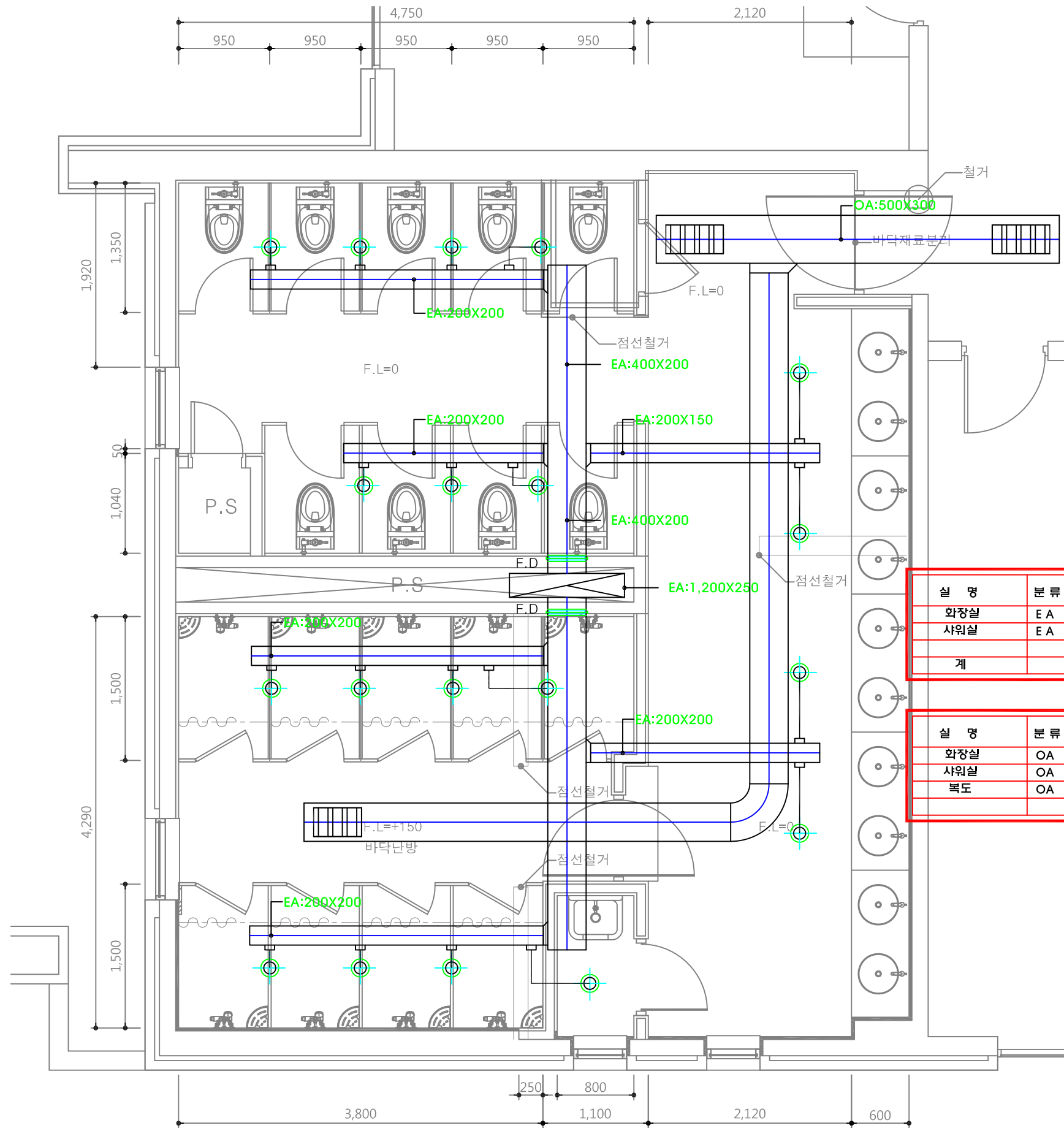
2,3,4층 화장실 확대 환기덕트 평면도(서북측) 축척 = (A1) 1/25 (A3) 1/50
